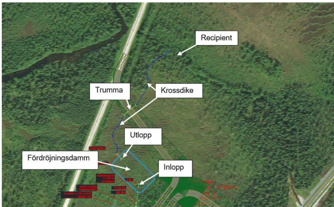
Figur 18. Förslag till dagvattenanläggningar samt utlopp i Koijuvaaranjoki. Koijuvaaranjoki mynnar i Leipojoki strax väster om utsläppspunkten, på andra sidan Nattavaaravägen. Figur från Sweco (2023).
