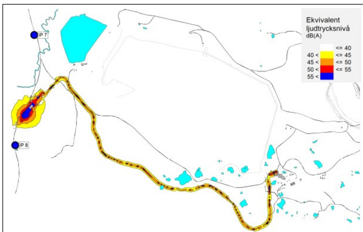
Figur 21. Beräknade ekvivalenta nivåer från nya bangården.
